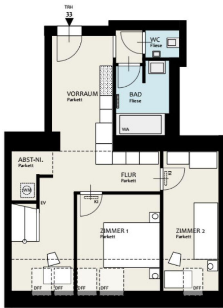
GRUNDRISS 1. DACHGESCHOSS
